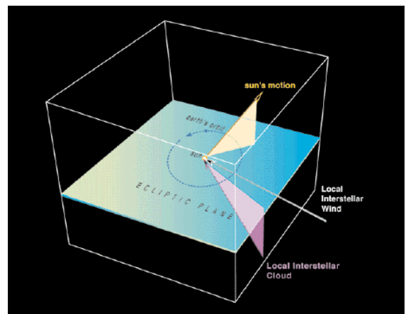
Рисунок 2. Относительные движения Солнца (желтая линия) и местного межзвездного облака (фиолетовая линия). Получившееся в результате относительное движение местного межзвездного ветра показано белой линией.
