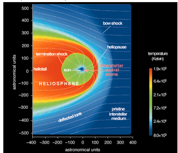
Рисунок 6. Солнечный ветер, истекающий из солнечной короны, заполняет пространство вокруг Солнца, называемое гелиосферой и взаимодействует с межзвездным газом. Заряженные частица (белые линии) в большинстве ионы водорода, отражаются границей гелиосферы, а нейтральные частички (розовые дуги), в основном атомы гелия и водорода, проникают в гелиосферу. Солнечный ветер, дующий от Солнца, показан белыми линиями внутри гелиосферы. В результате взаимодействия с межзвездным газом он формирует «гелиевый хвост», тянущийся за Солнечной системой.
